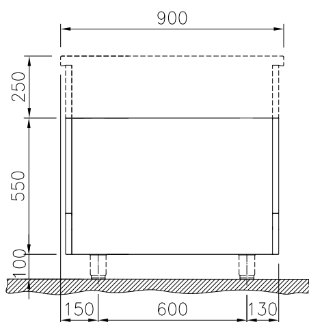
Boven aanzicht
